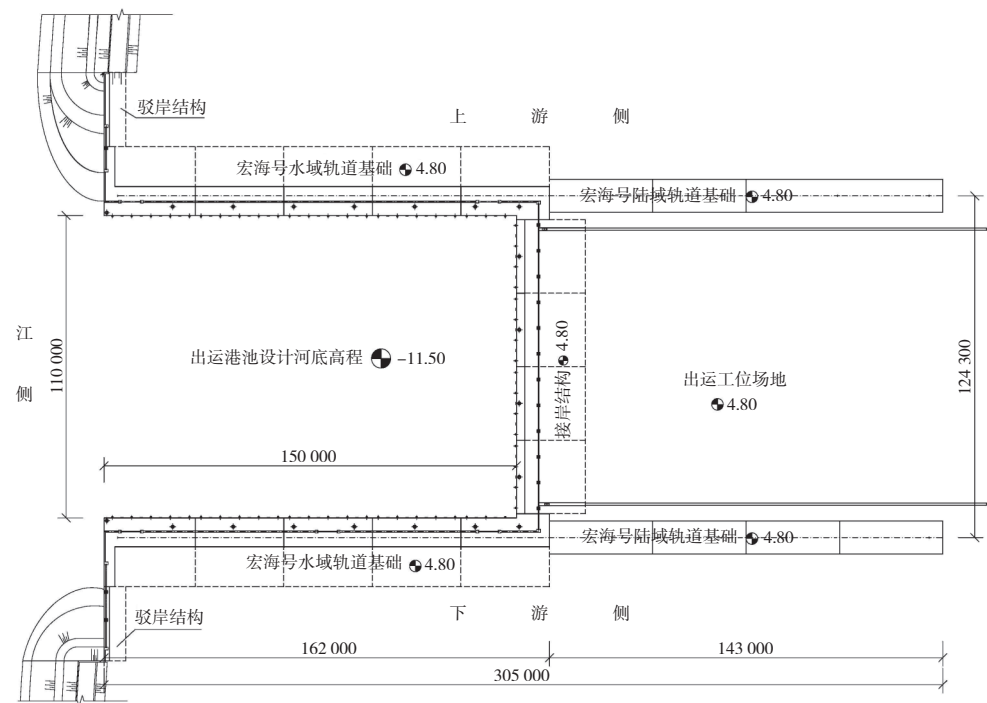
图2 出运码头平面布置
