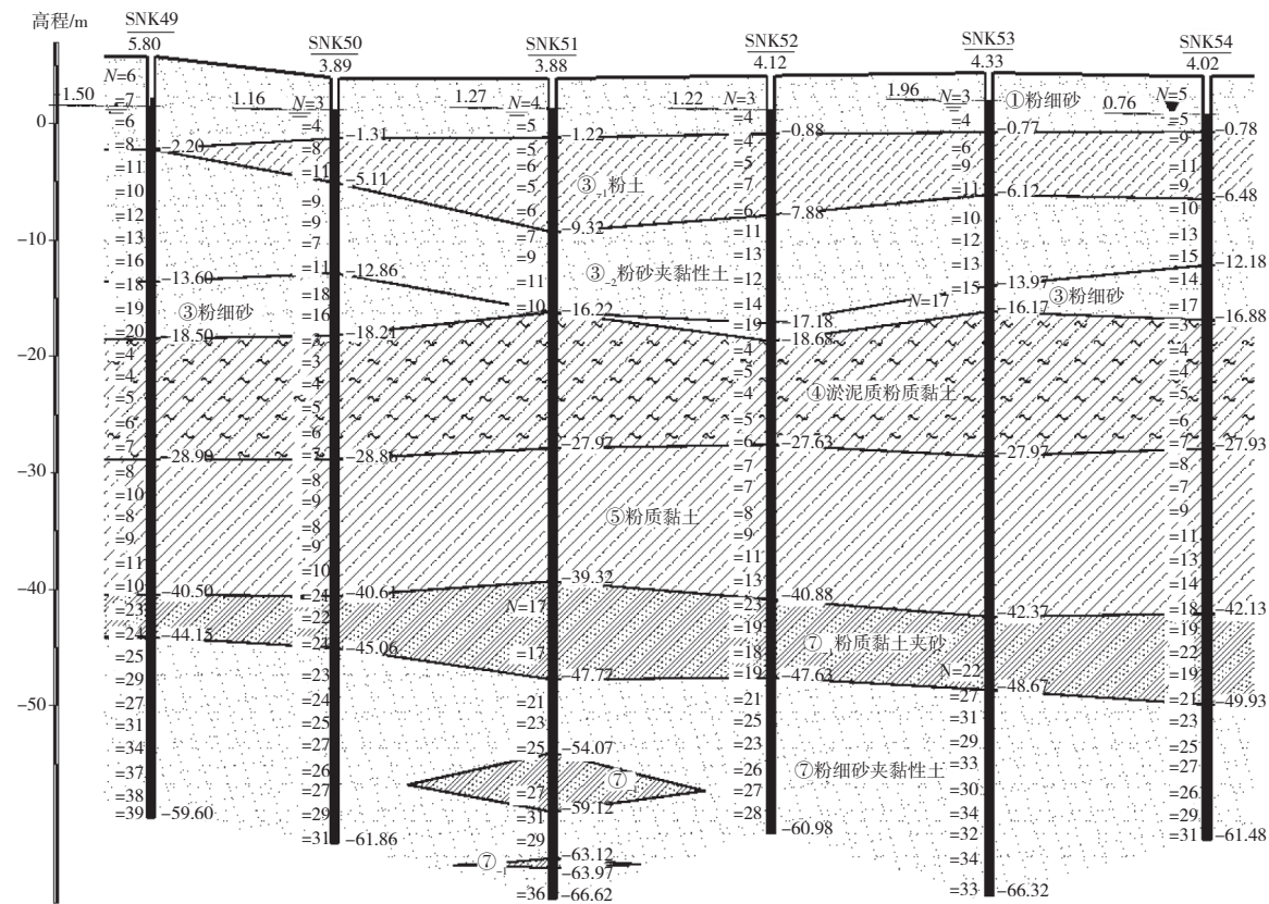
图3 工程地质典型断面
