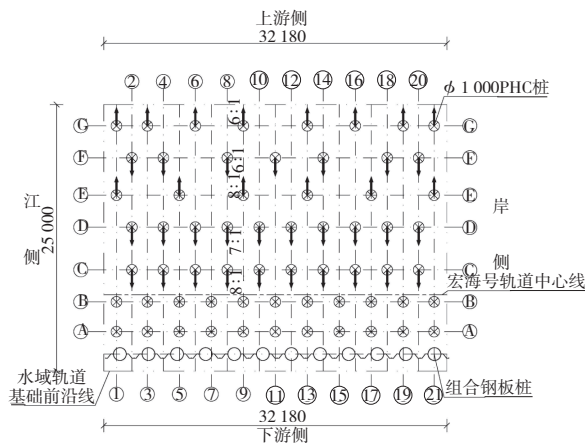
图5 结构分段桩位布置
