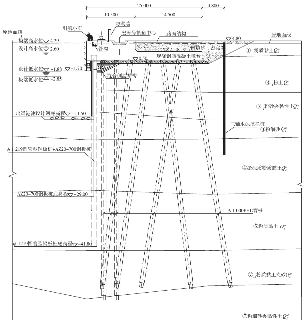
图4 码头结构典型断面
