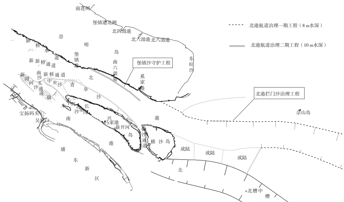
图3 北港航道分期治理方案
