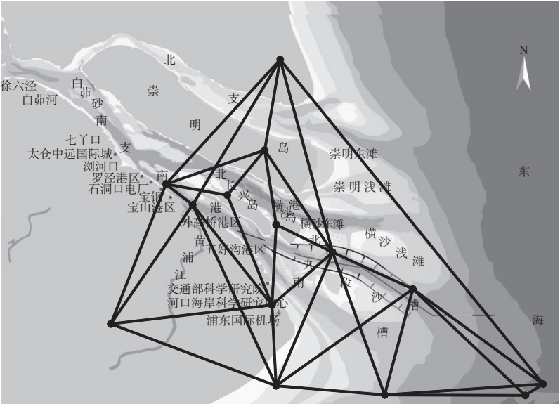
图7 GPS控制网布置
