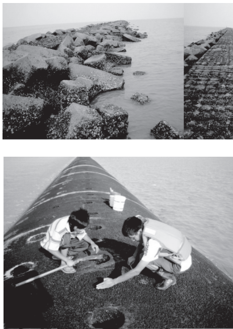
图12 利用丁坝和导堤建立的人工牡蛎礁
