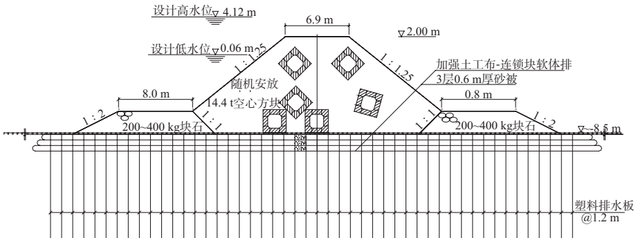
图6 空心方块斜坡堤典型断面
