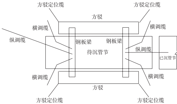
图5 双驳抬吊法沉放管节示意图
