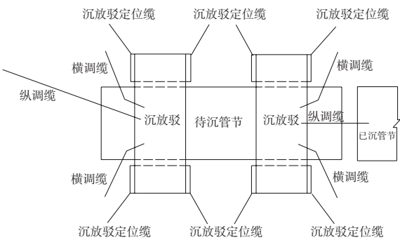
图6 双壳体船抬吊法沉放管节示意图
