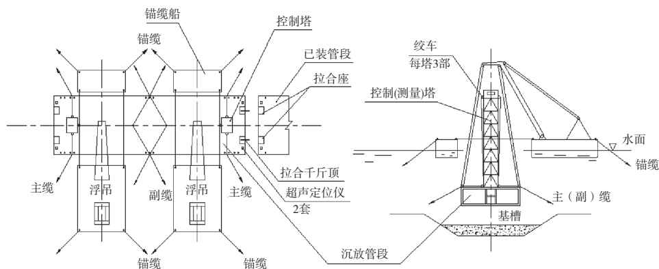
图1 双浮吊管节沉放示意图
