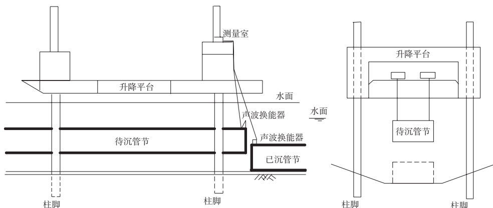
图3 升降平台法沉放管节示意图
