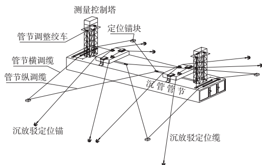
图2 浮箱法管节沉放示意图
