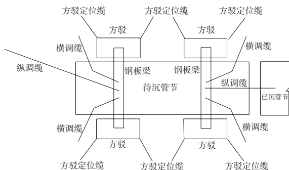
图4 四方驳抬吊法沉放管节示意图
