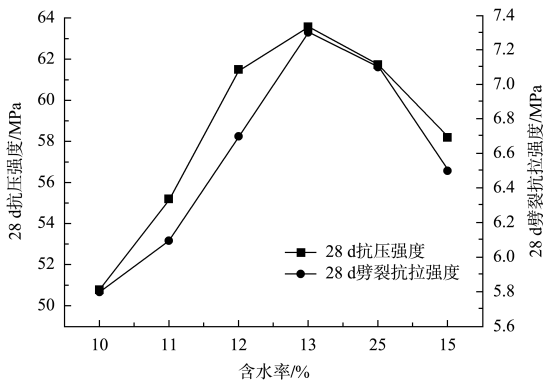
图 4 不同含水率下试件的强度 Fig. 4 Strength of specimens at different moisture contents
