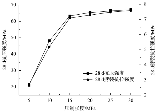
图 3 不同压制强度下试件的强度 Fig. 3 Strength of specimens under different compressive strengths
