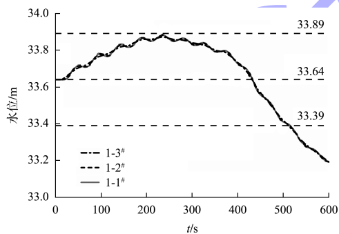
图9 一线船闸5 min旁侧泄水二线船闸下闸首附近水位过程线
