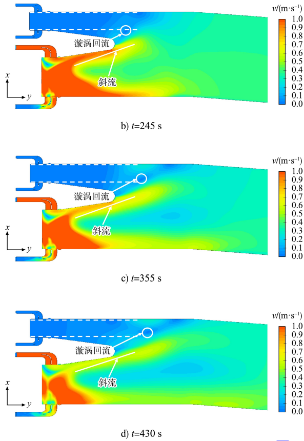
图7 一线船闸5 min左廊道单边泄水各典型时刻 出水口附近流速分布
