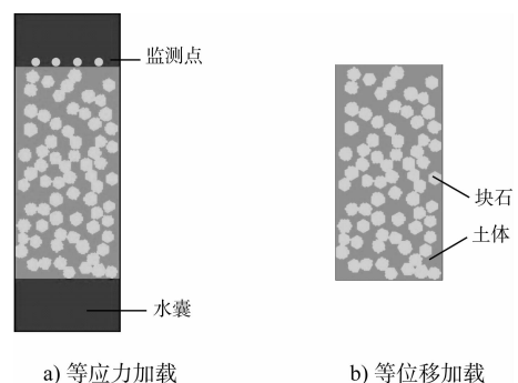
图5 等应力加载及等位移加载模型
