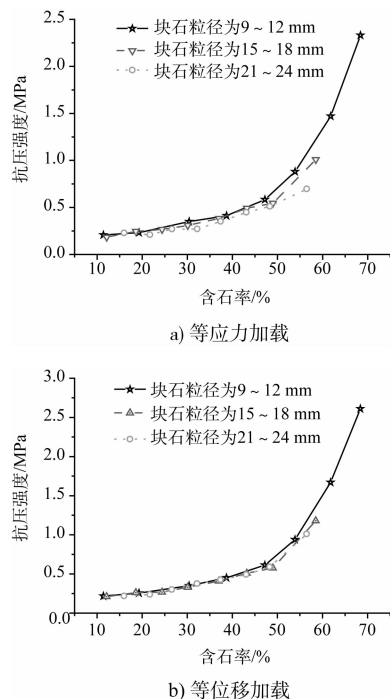
图10 不同加载情况下的含石率与抗压强度关系曲线
