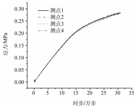
图 6 土石混合体顶端竖向应力的监测曲线
