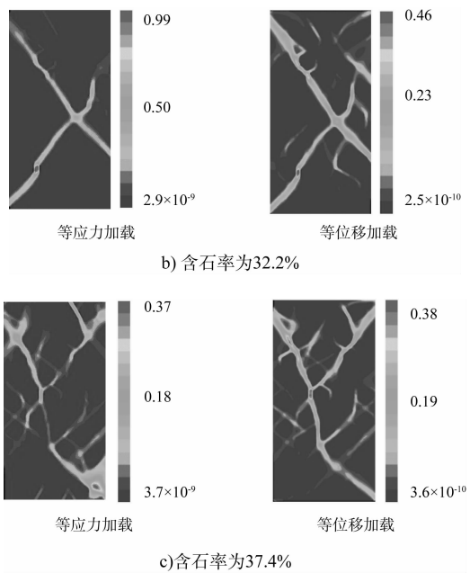
图9 两种加载方式下不同含石率的土石混合体内部的塑性剪应变云图
