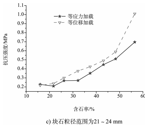
图8 不同粒径土石混合体的强度随含石率的变化曲线
