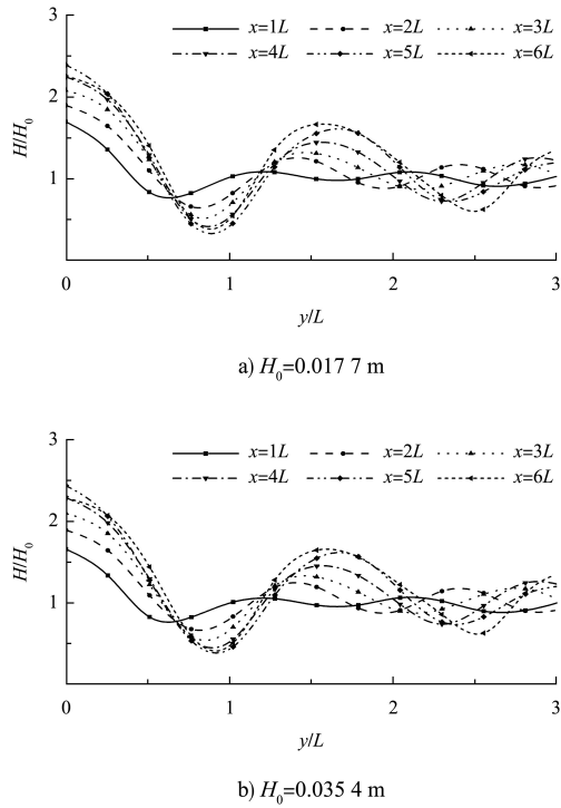
图 11 垂直墙面方向比波高分布特征 ( \varphi_i = 20^\circ , x = 1L \sim 6L )
