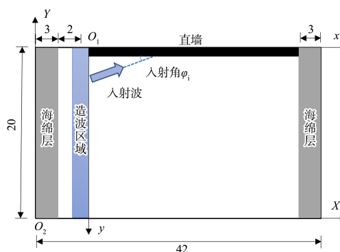
图 2 计算域 (单位: m)
