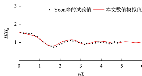
b) Stem波垂直墙面方向比波高分布
