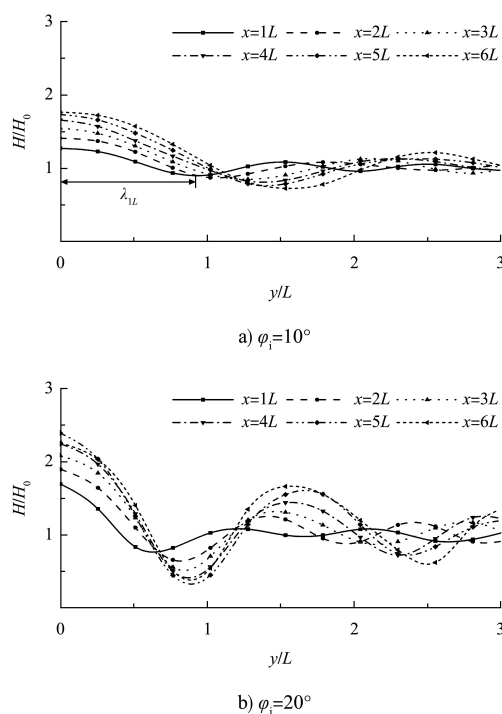
图 7 垂直墙面方向比波高分布特征 ( H_0 = 0.0177 m, x = 1L \sim 6L )
