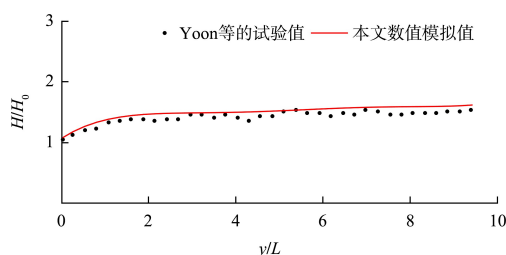
a) Stem波沿墙方向比波高分布
