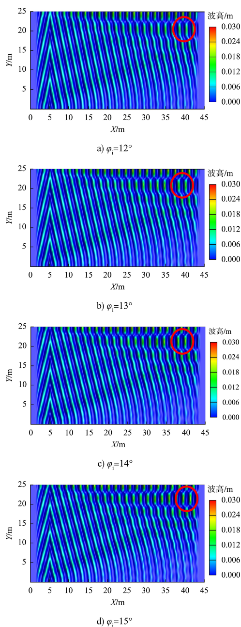
图 5 不同入射角下瞬时自由表面等值线
