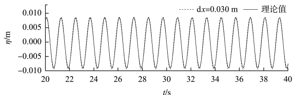
图 4 波面历时曲线
