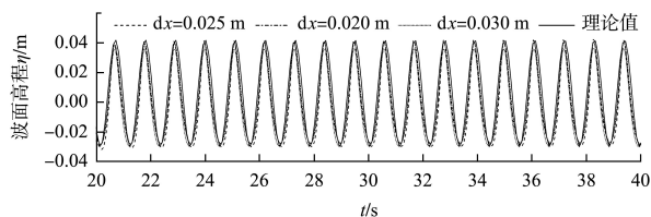
图 1 网格收敛性验证结果
