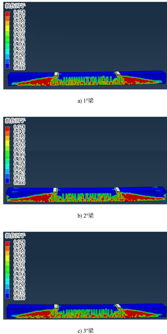
图 6 1#、2#及3#梁受拉损伤因子云图
